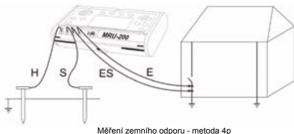
Měření zemního odporu - metoda 4p
